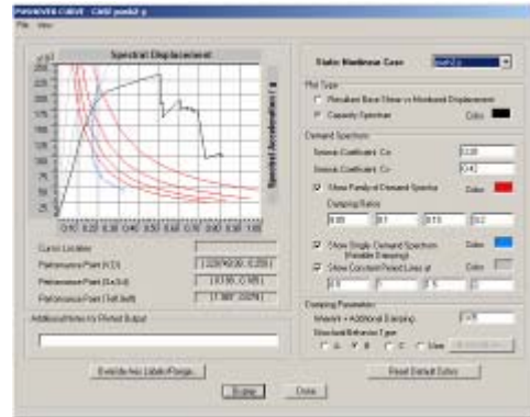
Gambar 20. Arah Y, \delta_T = 0.250 m
