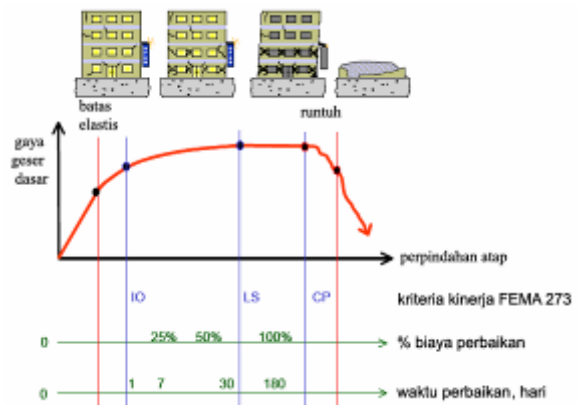
Gambar 1. Ilustrasi Rekayasa Gempa Berbasis Kinerja (ATC58)
