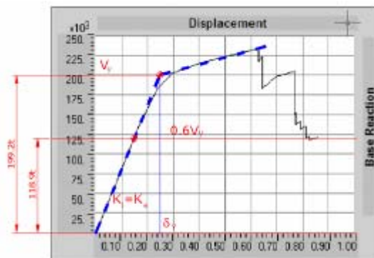
Gambar 18. Kurva Bi-linier Pushover Arah-Y
